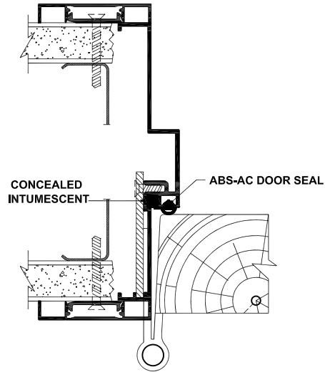
B DOOR FRAME HINGE JAMB
